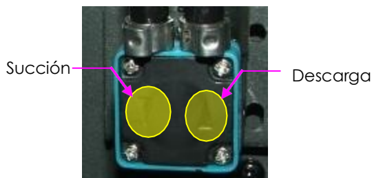
flecha de la cabeza
