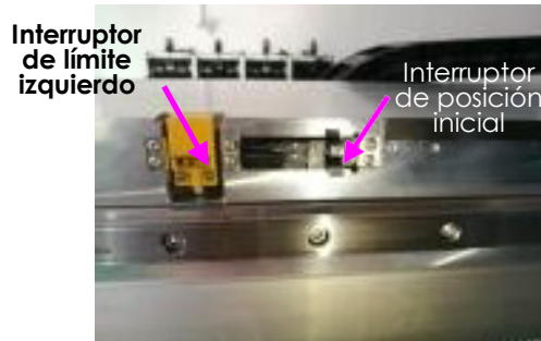
Interruptores de límite del extremo izquierdo
